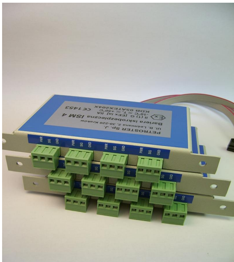
Rysunek 4: Moduł bariery iskrobezpiecznej.
