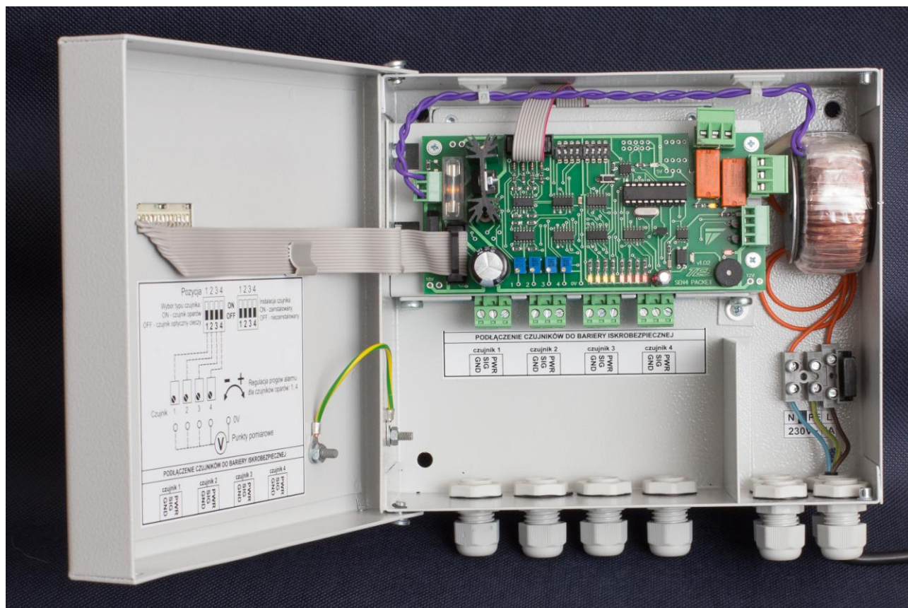
Rysunek 2: Widok wnętrza centrali Tank Ranger model 5.
