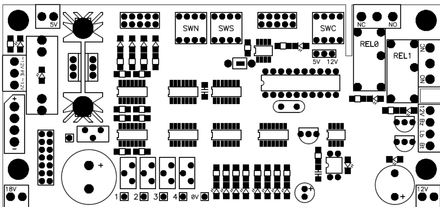
Rysunek 3: Płyta główna centraliki Tank Ranger model 5.
