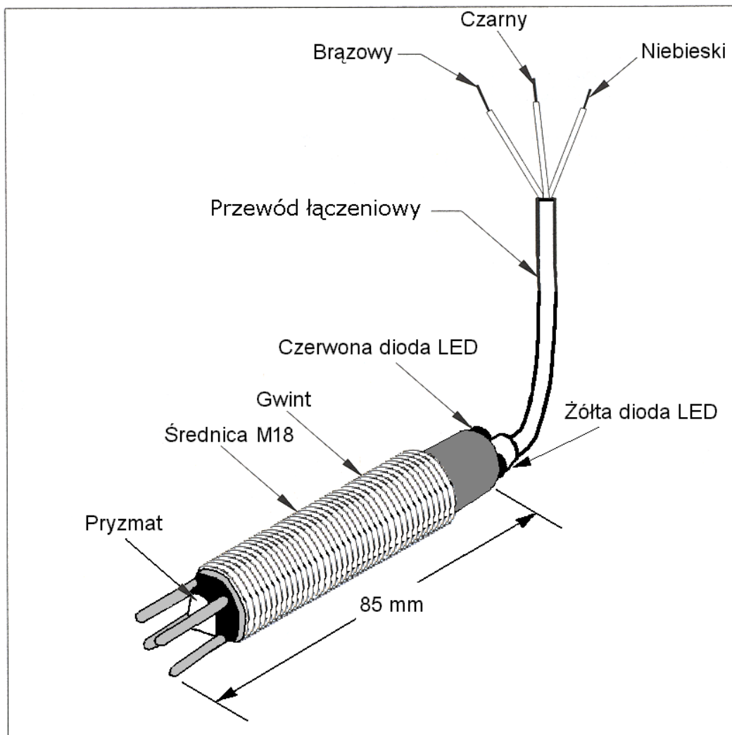
Rysunek 13: Selektowny czujnik optyczny cieczy PCOpt/s.
